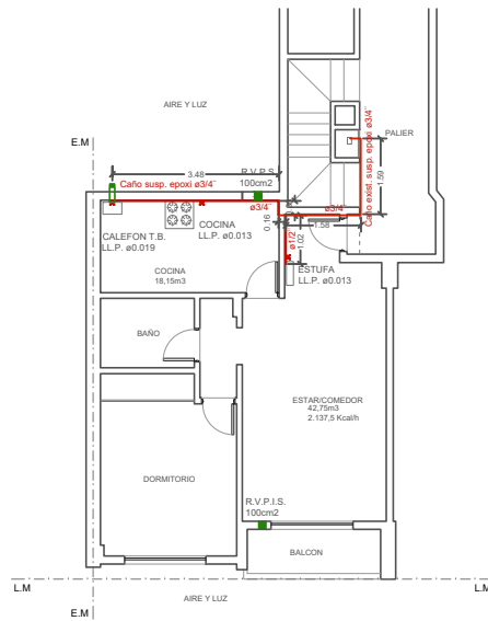
PLANTA U. 01-04 Esc: 1:100
